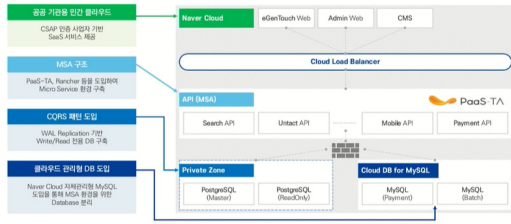
(그림 3) OO시 도서관의 SaaS 클라우드 사용 예 (Figure 3) The SaaS based OO Library Case
